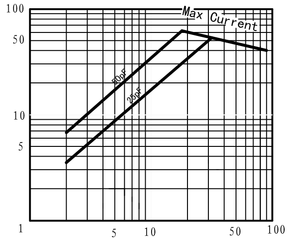
频率曲线 (MHz) U_{pw}=15kV
