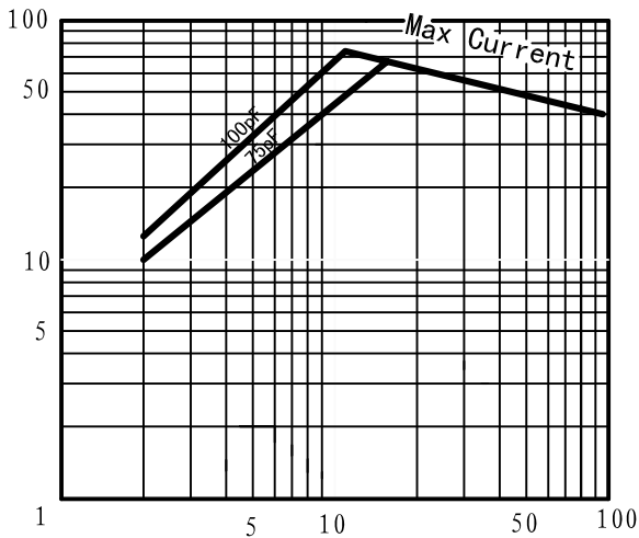
频率曲线 (MHz) U_{pw}=15kV
